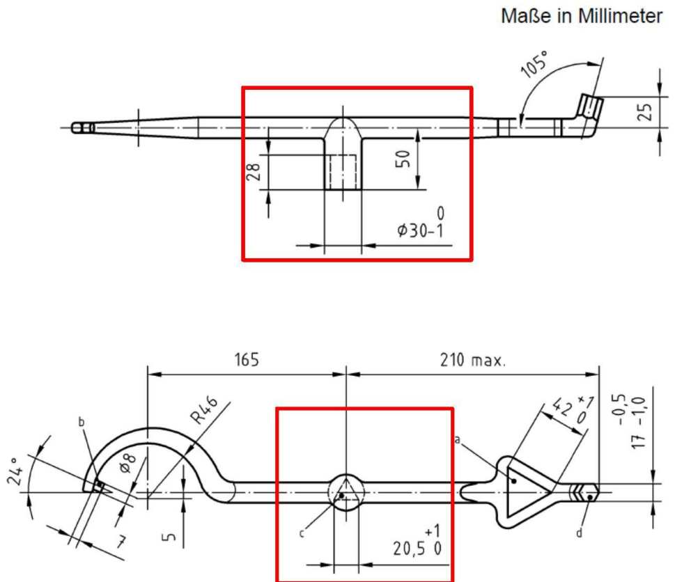
Abbildung 2 Überflurhydrantenschlüssel
