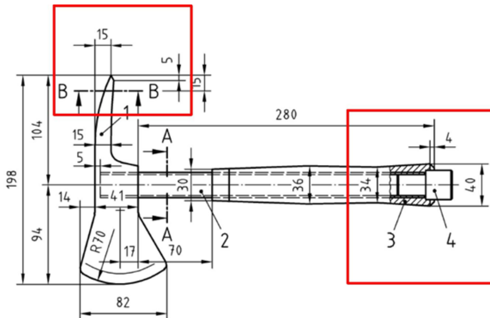
Abbildung 5 Feuerwehrbeil
