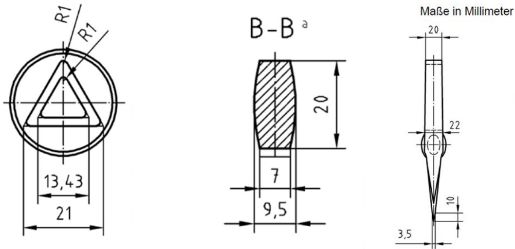
Abbildung 6 Bemaßungen Feuerwehrbeil
